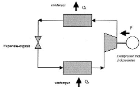
Figuur 1 Kringloopkoelmachine
